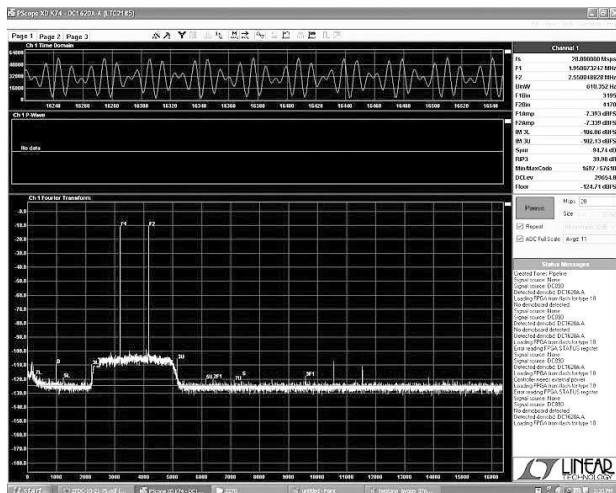
Рисунок 3. Двухтональный спектр LTC2270. Повышенный уровень шумов привнесен генератором сигналов.
