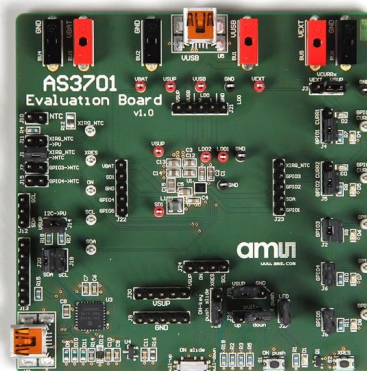
Оценочная плата для AS3701.
