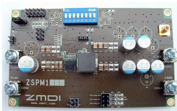
Оценочный набор ZSPM15xx-KIT01
