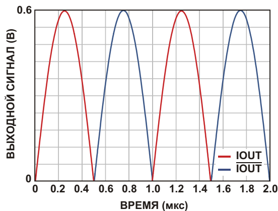
Рисунок 6. Размах напряжений на выходах I_{OUT} и \bar{I}_{OUT} микросхемы AD9834C. Артефакты, обусловленные наложением частот, не показаны.
