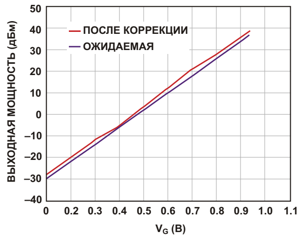
Рисунок 14. Выходная мощность схемы при использовании ФНЧ пятого порядка (частота среза 20 МГц). Частота сигнала равна 14.0956 МГц.
