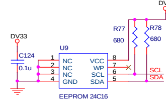
EEPROM 24C16
