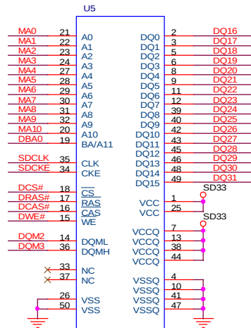
ESMT M12L16161A-?
