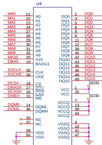
ESMT M12L16161A-?
