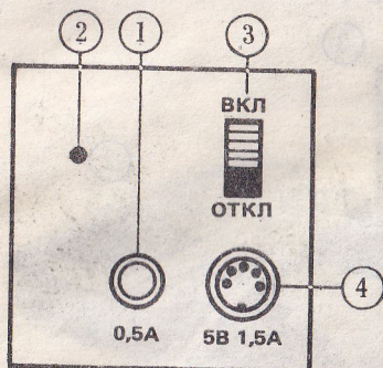
Рис. 4 Блок питания (вид спереди):
