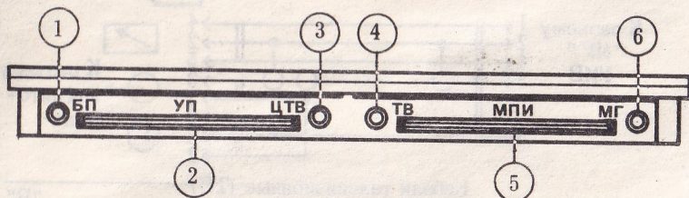
Рис. 3 Вид панели УИВ (со стороны внешних разъемов):
